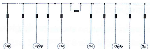
Rys.1. Konfiguracja maksymalna GPZ/RPZ
